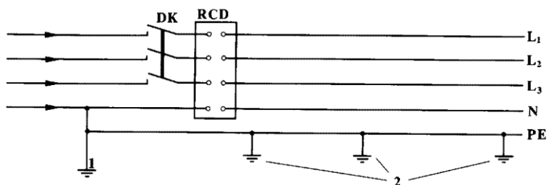
图5.1.2 三相四线供电时局部TNS接零保护系统保护零线引出示意图
